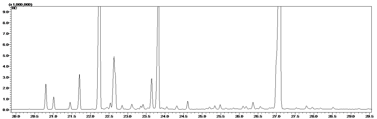
▲天然廣藿香精油GC-MS圖譜驗證
